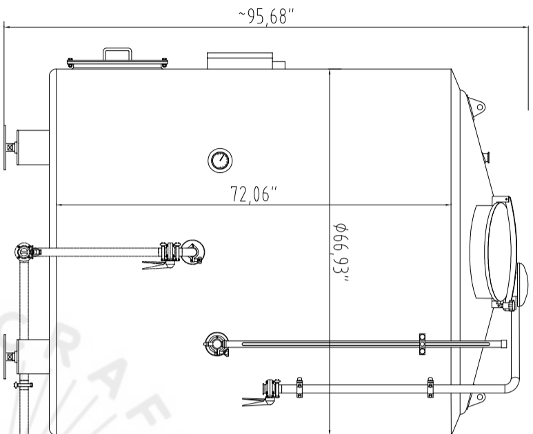
15BBL HLT
