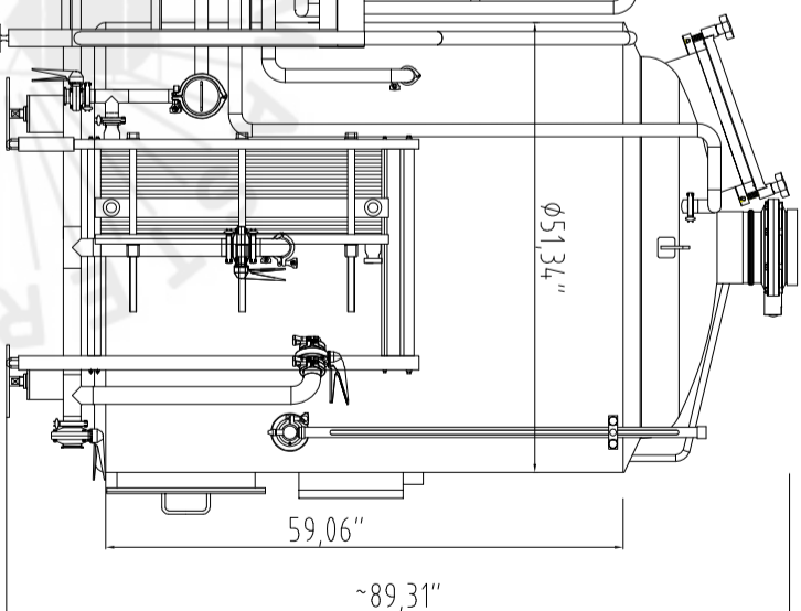
7BBL KW(F)
