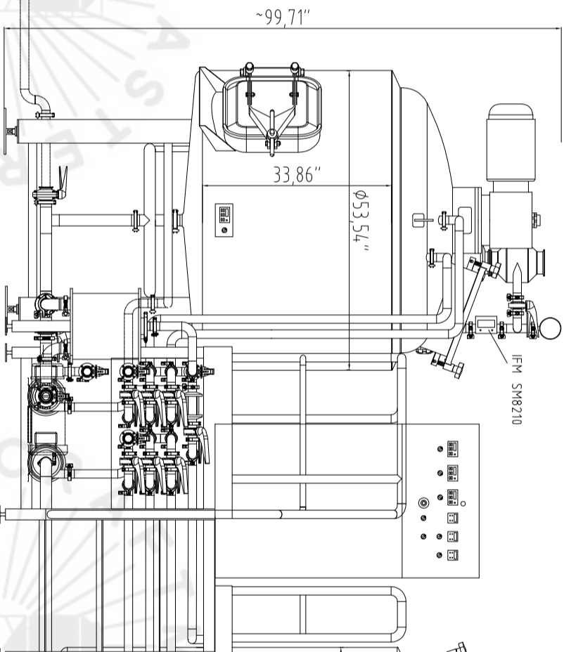
7BBL MLT
